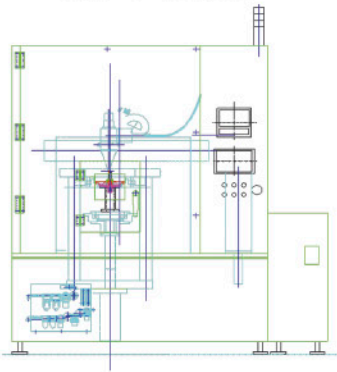
各種レーザー溶接用治具
