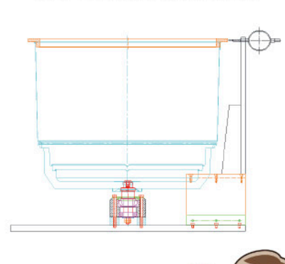
大型ドラム形状製品回転振れ検査治具
