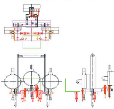
製品組付け高さ簡易検査治具
